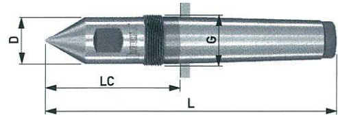
Form 255 similar to DIN 807, 60°
