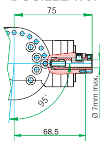
BROCHE BMR 10 DOUILLE W07-11-38
