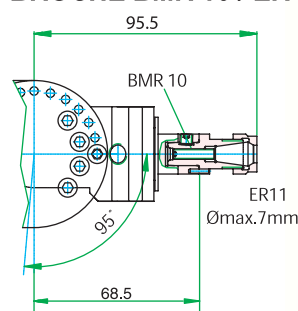
BROCHE BMR 10 DOUILLE W07-11-38
