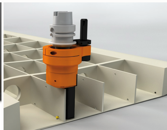
Exemple d'usinage sur une aile d'avion Machining on a airplane wing
